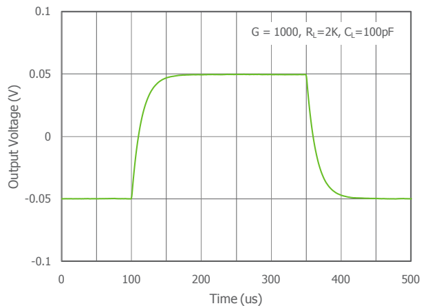
小信号脉冲响应 ( G = 1000 )
