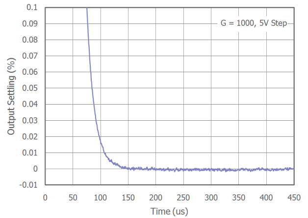
大信号建立时间 ( G = 1000 )
