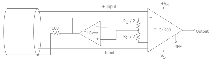
图 1: 共模屏蔽驱动器
